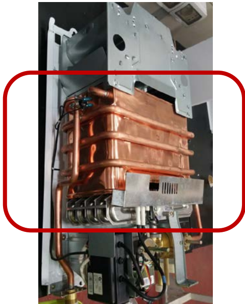
Бескислородный медный теплообменник
