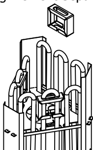
Разделитель нагревательных элементов Heating Element Separator
