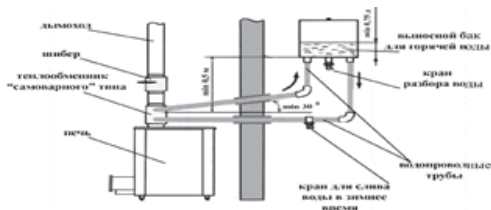
Схема подключения подачи горячей воды через теплообменник самоварного типа
