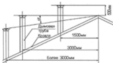
Расчёт высоты дымохода над крышей
