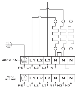
Kuva 2. Kytentäkaavio
