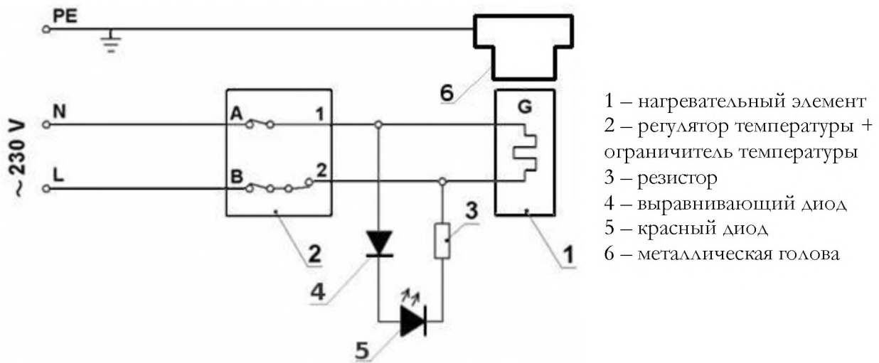
Рис. 2 Схема электрической сети
