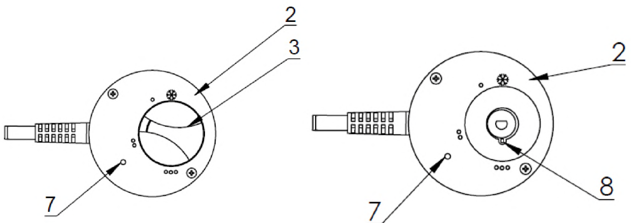
Рис.1 Конструкция нагревательного элемента.
