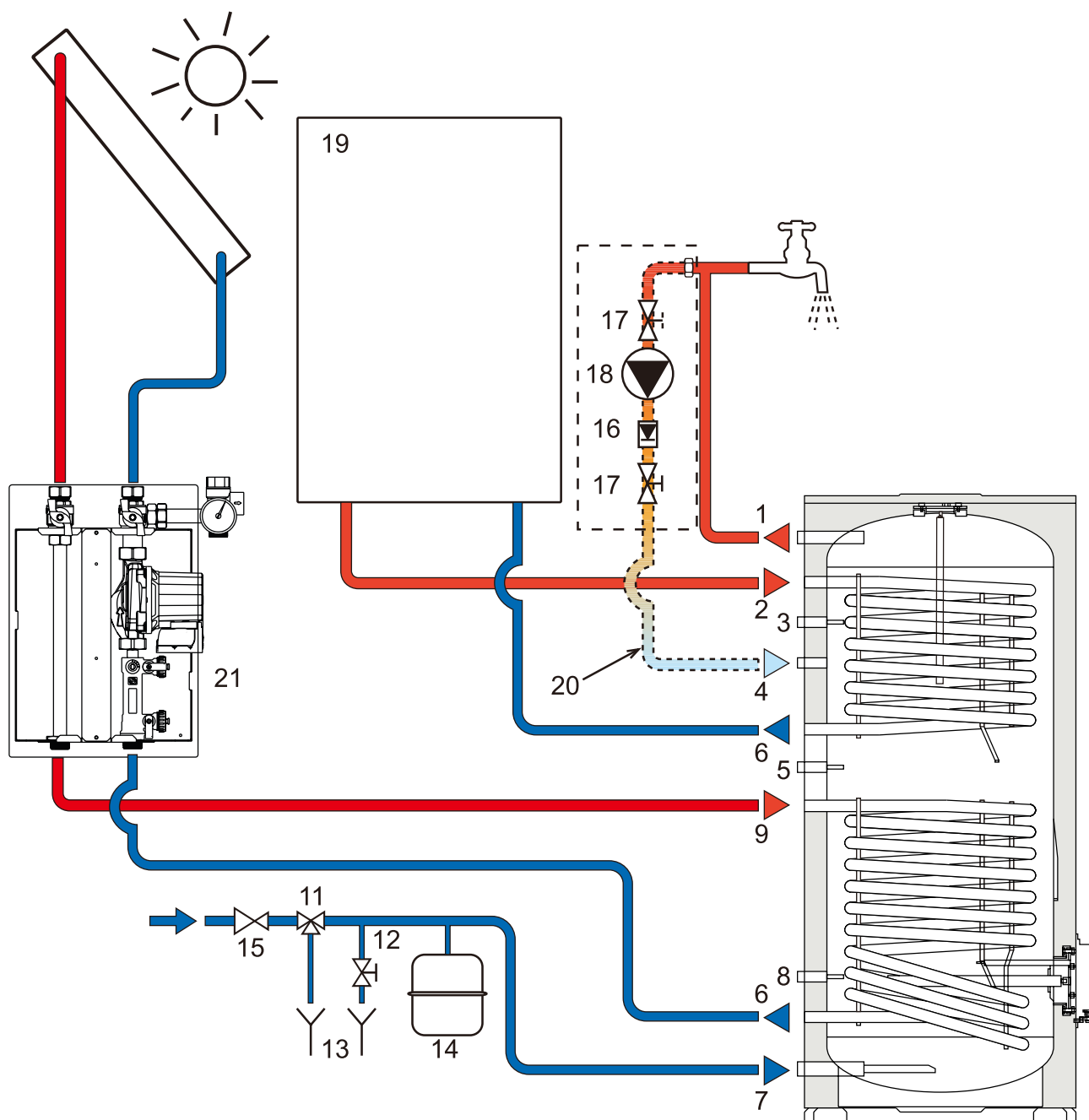
Рис. 6 – Гидравлический контур ECOUNTIT F 2C
