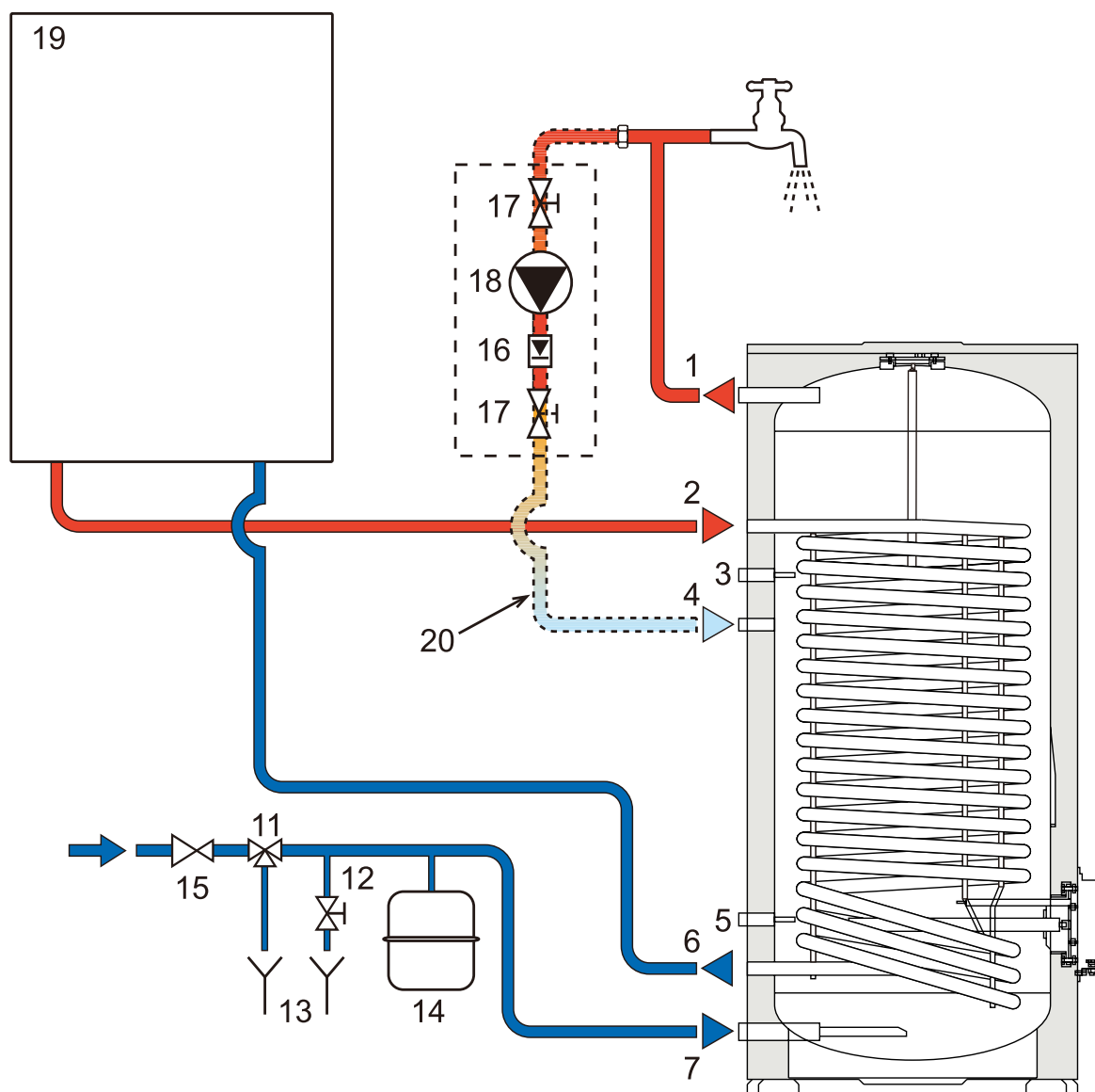
Рис. 5 – Гидравлический контур ECOUNT F 1C
