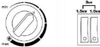
Мал.3 Панель керування моделі BRICK 3: Перемикачі режимів (ліворуч). Ручка регулювання термостата (праворуч).
