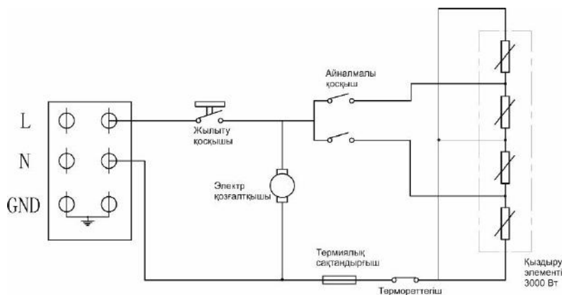
6-сур. Электр схемасы BRICK 3
