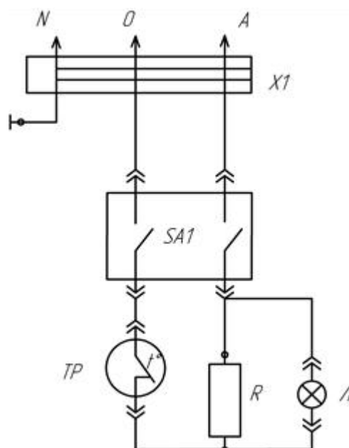
Рис. 2 Схема электрическая принципиальная
