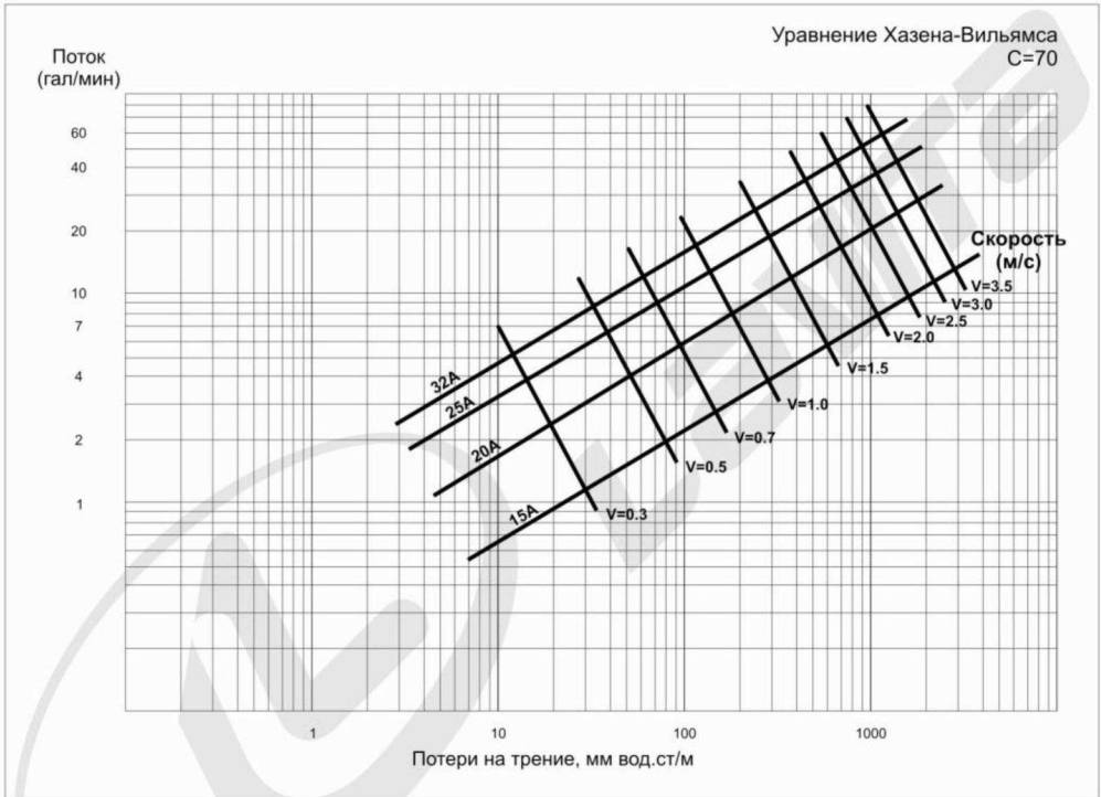
Рис.1 Гидравлические потери
