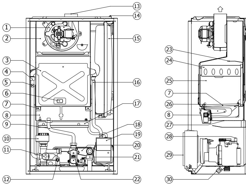
Рисунок 25. Компоненты котла
