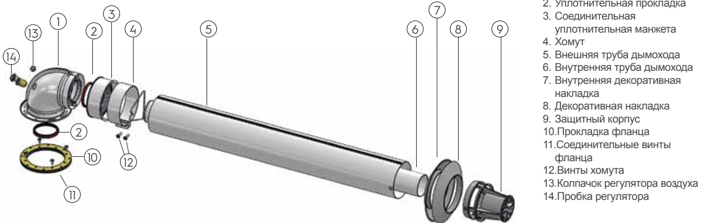
Рисунок 11. Дымоход котла
