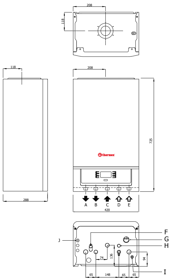
Рисунок 7. Размеры и подключения котла BaliusPlus
