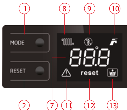
Рисунок 27. Экран автоматической панели управления Balius
