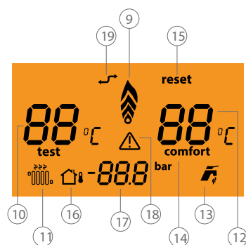
Рисунок 29. Экран автоматической панели управления BaliusPlus
