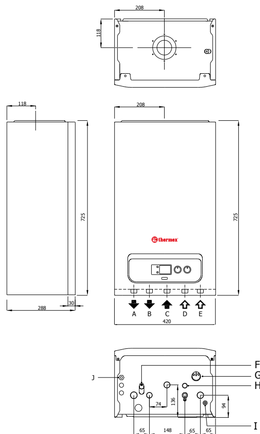
Рисунок 6. Размеры и подключения котла Balius
